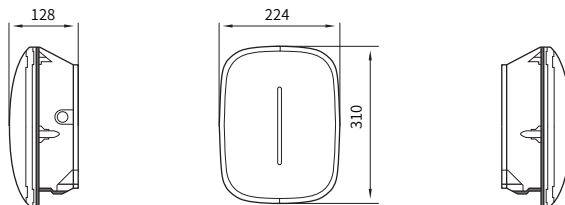
Рис 3.1 Внешний вид и размеры устройства
