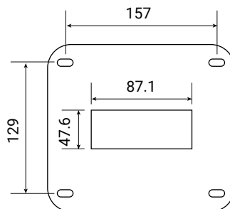
Рисунок 4.7 Разметка отверстий для установки анкерных болтов. Размеры в мм.
