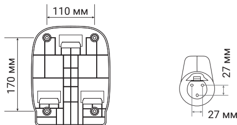
Рис. 4.1. Расположение отверстий
