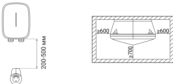
Рисунок 4.2 Схема настенной установки зарядного устройства
