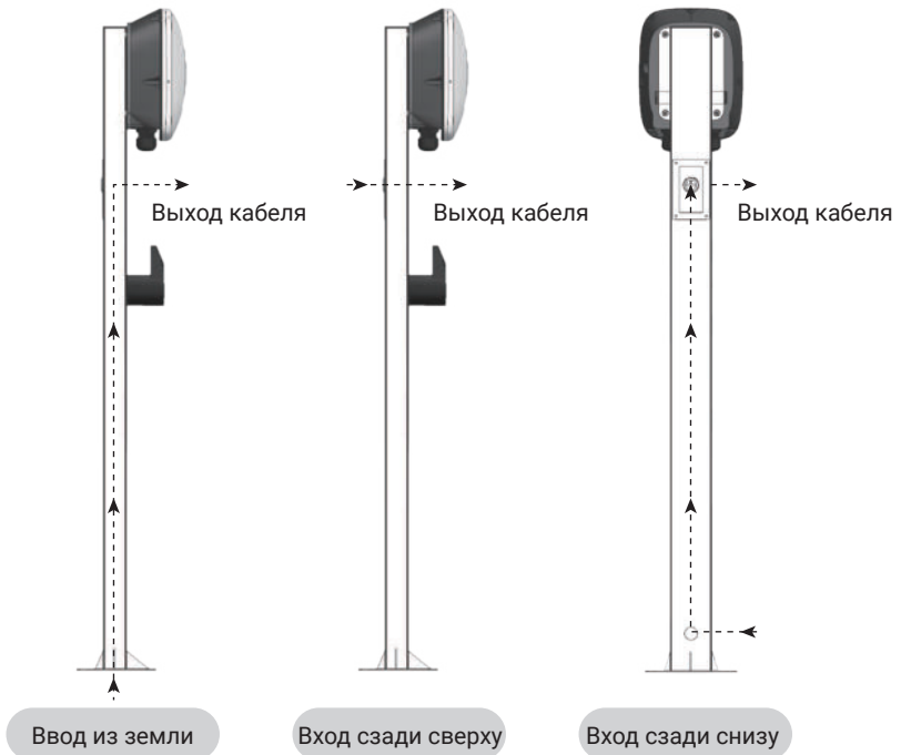
Рисунок 4.8 Варианты ввода кабеля
