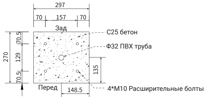
Рисунок 4.6 Основание стойки. Размеры в мм.
