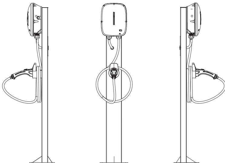
Рисунок 4.5 Схема установки зарядного устройства на стойку
